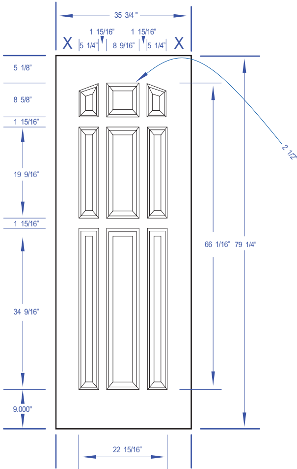
DOOR DIMENSIONS
