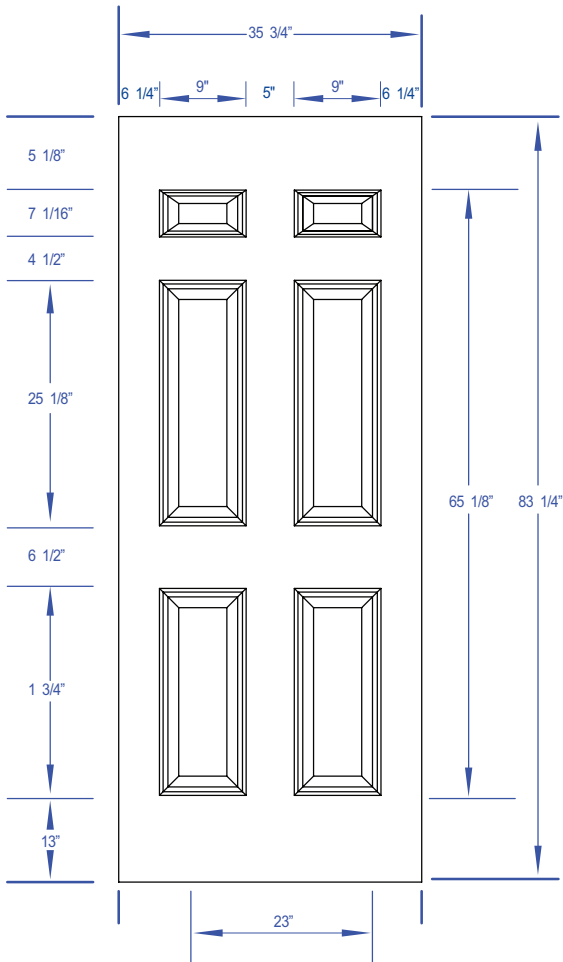
DOOR DIMENSIONS
