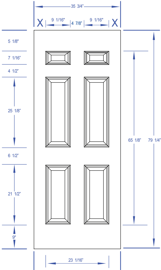
DOOR DIMENSIONS
