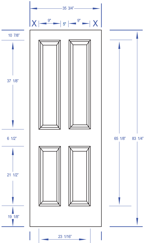
DOOR DIMENSIONS
