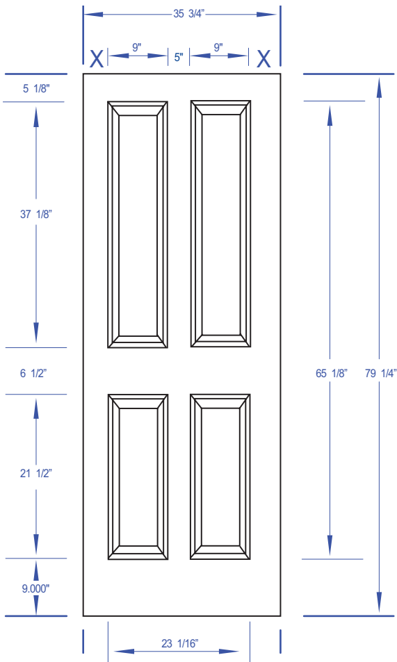
DOOR DIMENSIONS
