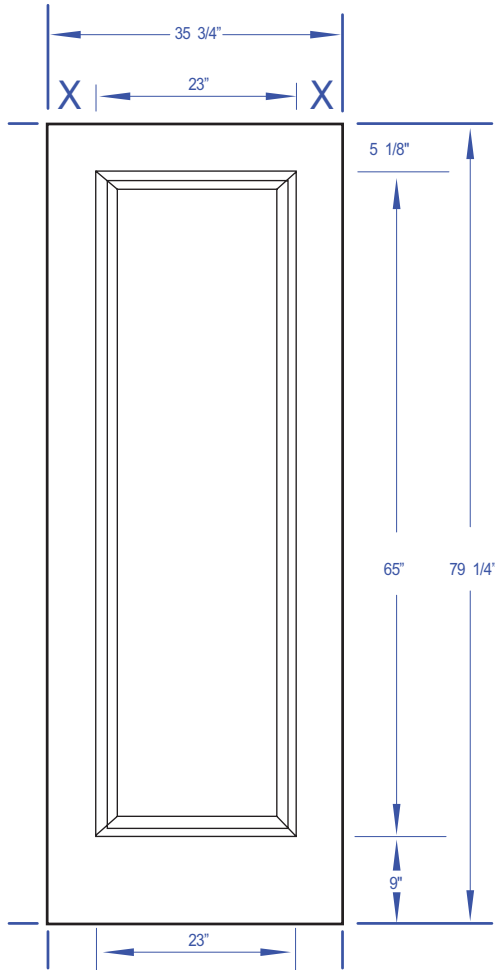
DOOR DIMENSIONS
