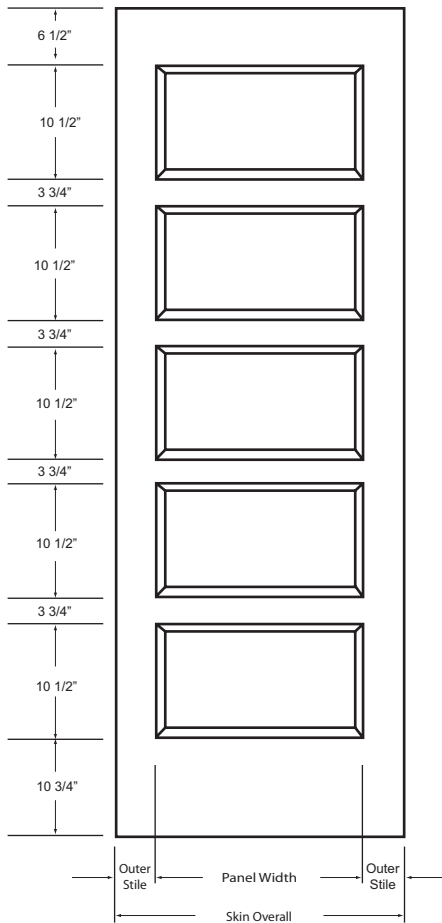
DOOR DIMENSIONS
