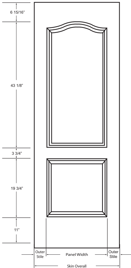
DOOR DIMENSIONS
