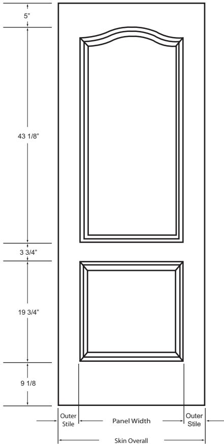
DOOR DIMENSIONS
