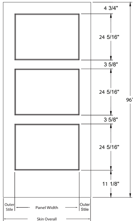
DOOR DIMENSIONS
