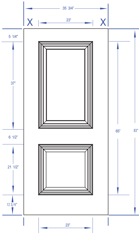
DOOR DIMENSIONS
