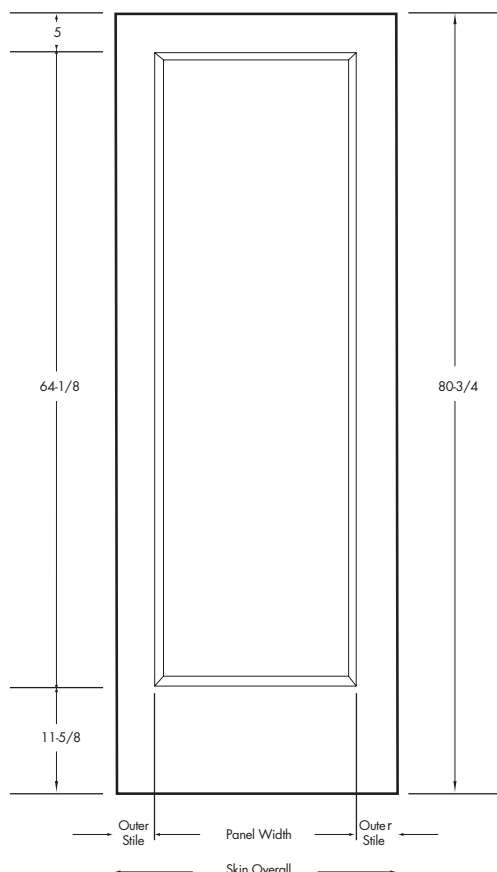
DOOR SKIN DIMENSIONS*
