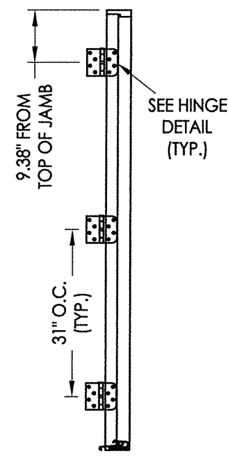
HINGE JAMB
