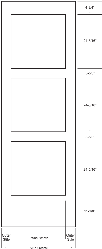
DOOR DIMENSIONS
