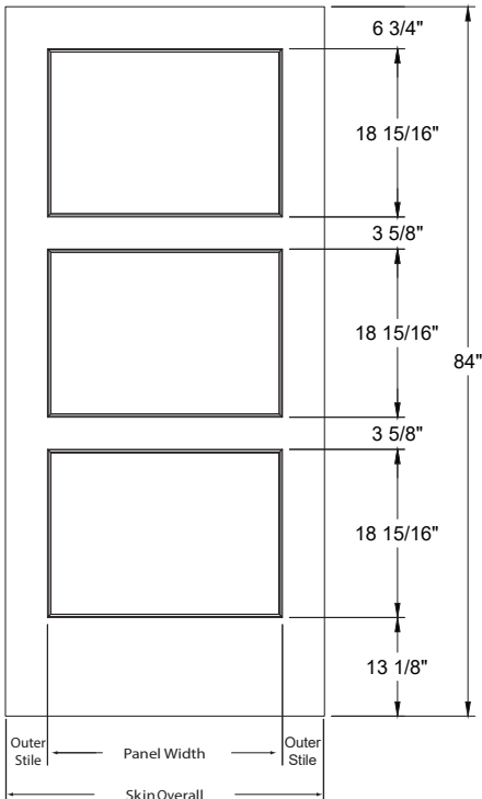
DOOR DIMENSIONS
