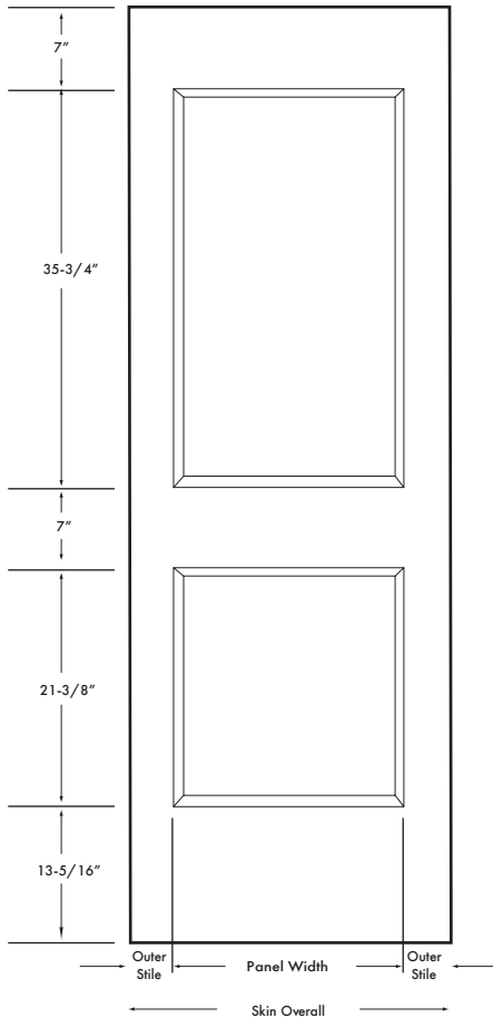
DOOR DIMENSIONS
